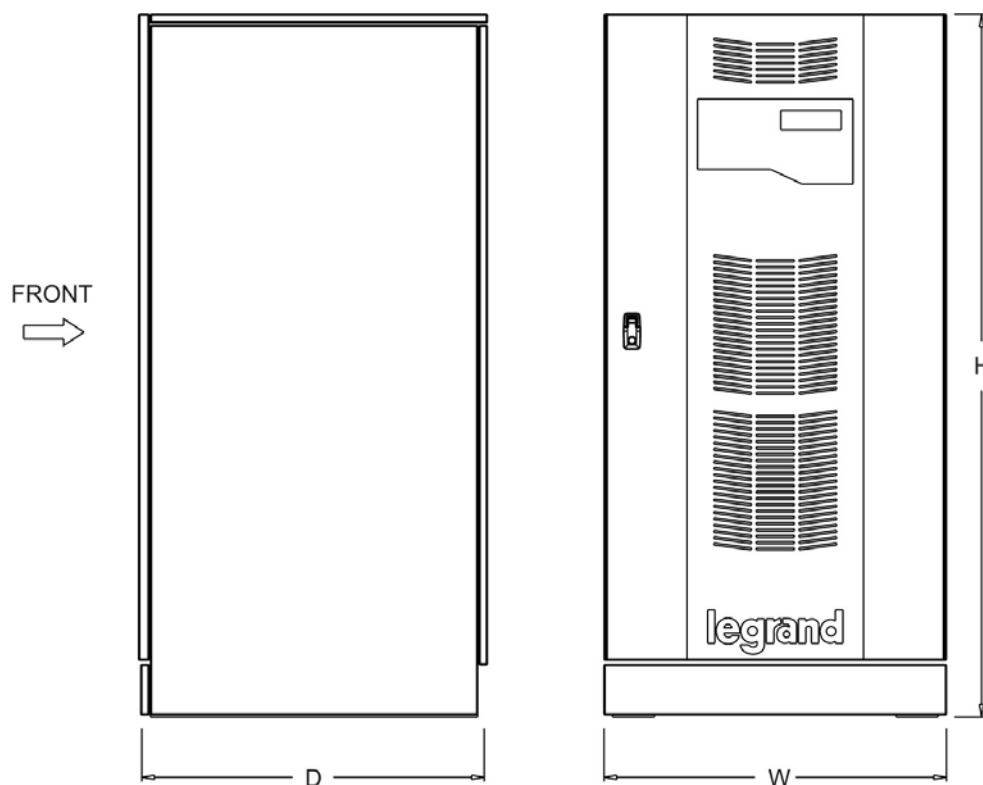
Figura 4 – Ingombri UPS KEOR HP
