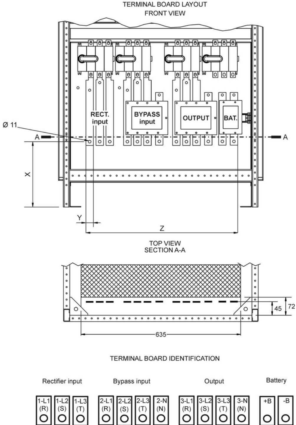
Illustration 6 – Position des bornes du KEOR HP
