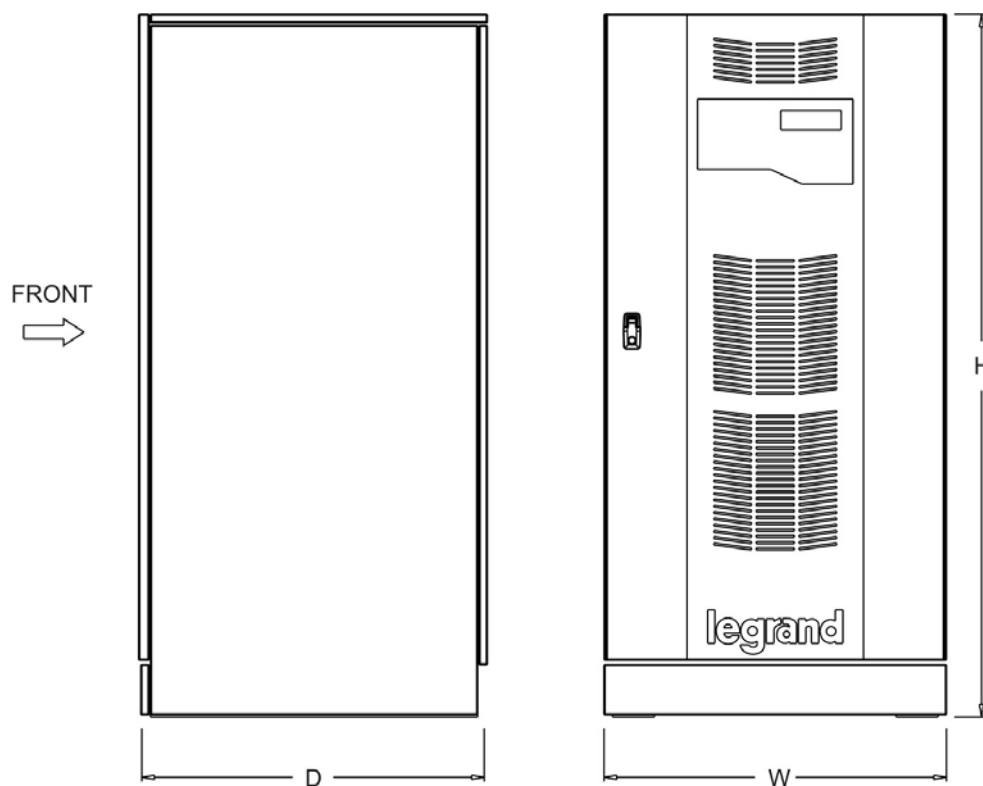
Illustration 4 – Dimensions totales de l'UPS KEOR HP
