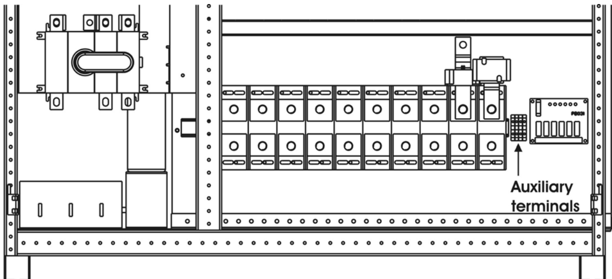
Illustration 7 – Position des bornes auxiliaires du KEOR HP
