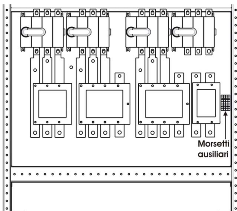
Figura 7 – Posizione morsetti ausiliari KEOR HP
