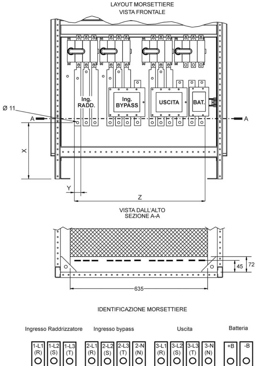
Figura 6 – Posizione morsetti potenza KEOR HP
