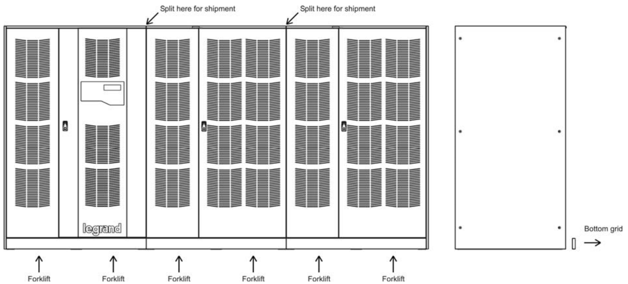
Illustration 4 – Maintenance de l'UPS KEOR HP 800 kVA
