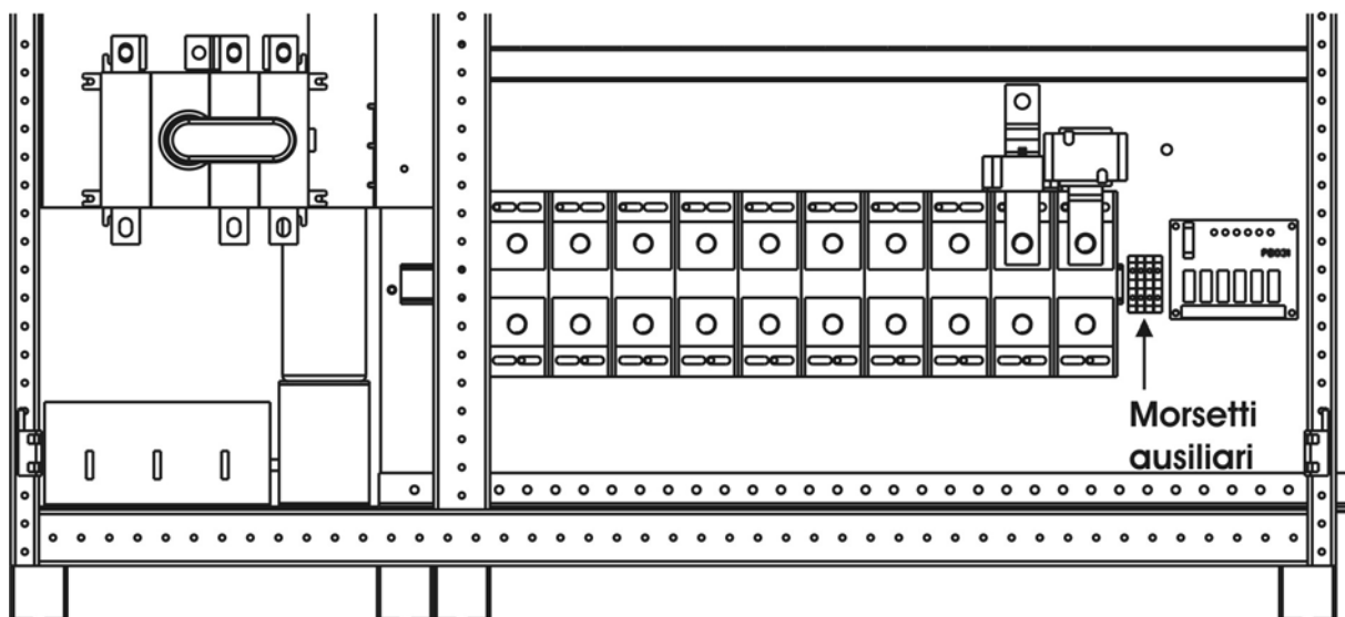
Figura 7 – Posizione morsetti ausiliari KEOR HP
