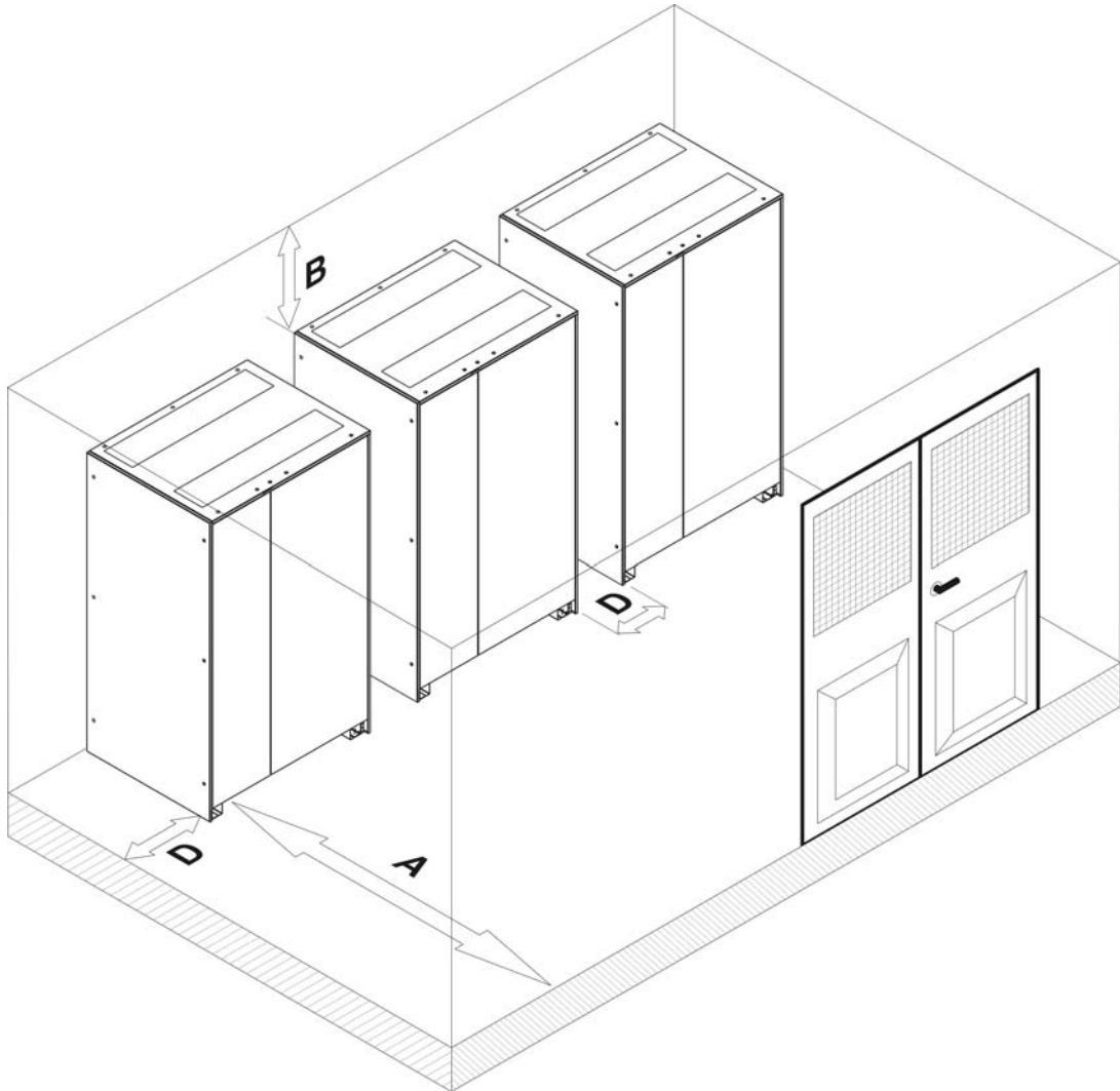
Illustration 5 – Dégagement minimum
