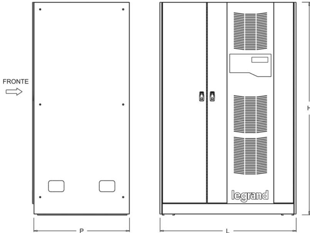
Figura 4 – Ingombri UPS KEOR HP
