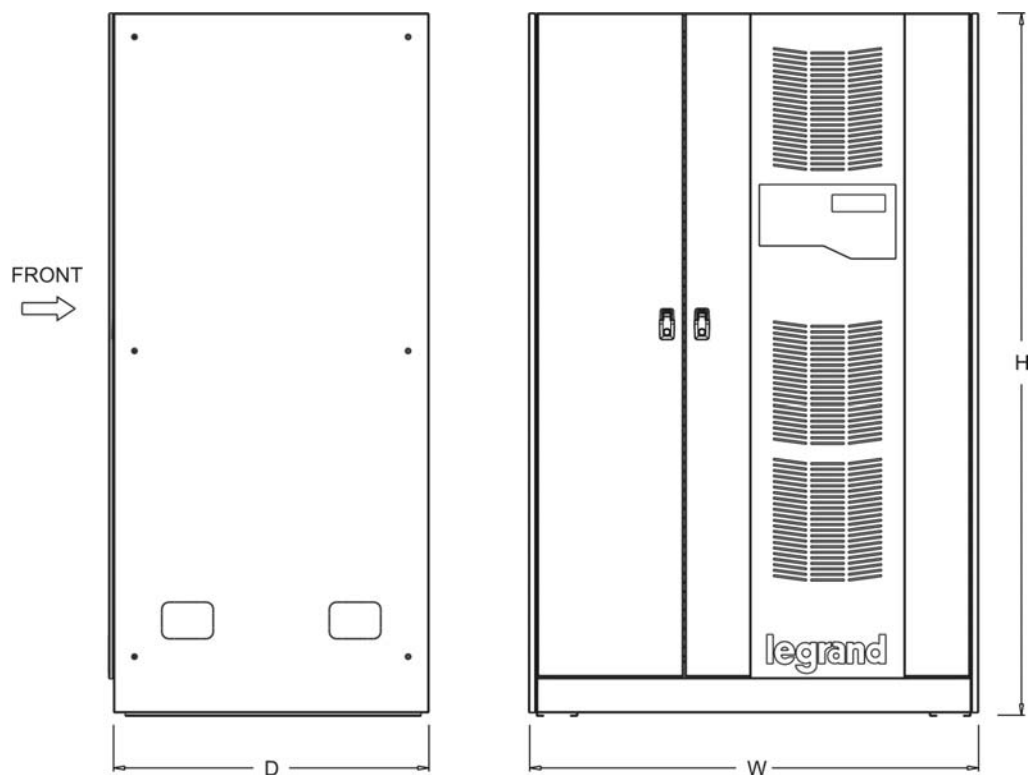
Illustration 4 – Dimensions totales de l'UPS KEOR HP
