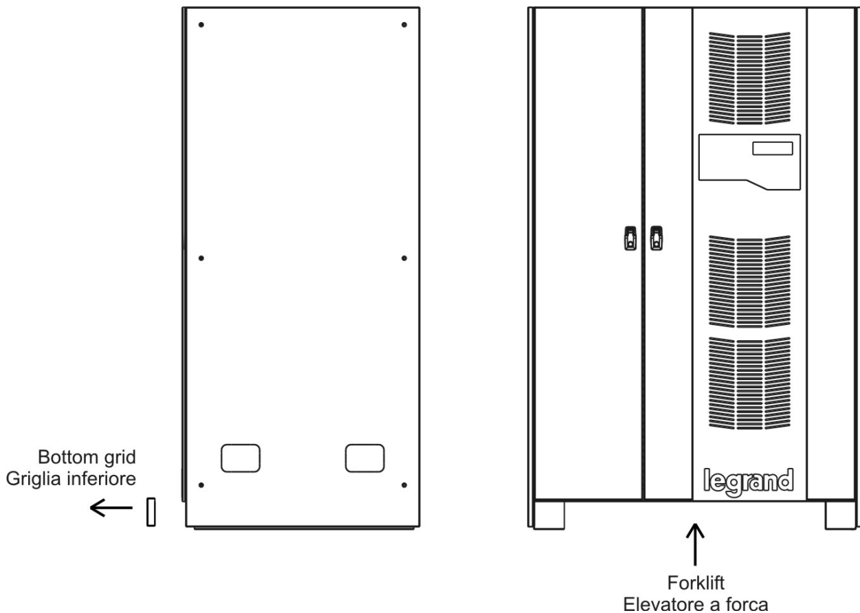
Figura 2 – Movimentazione UPS KEOR HP
