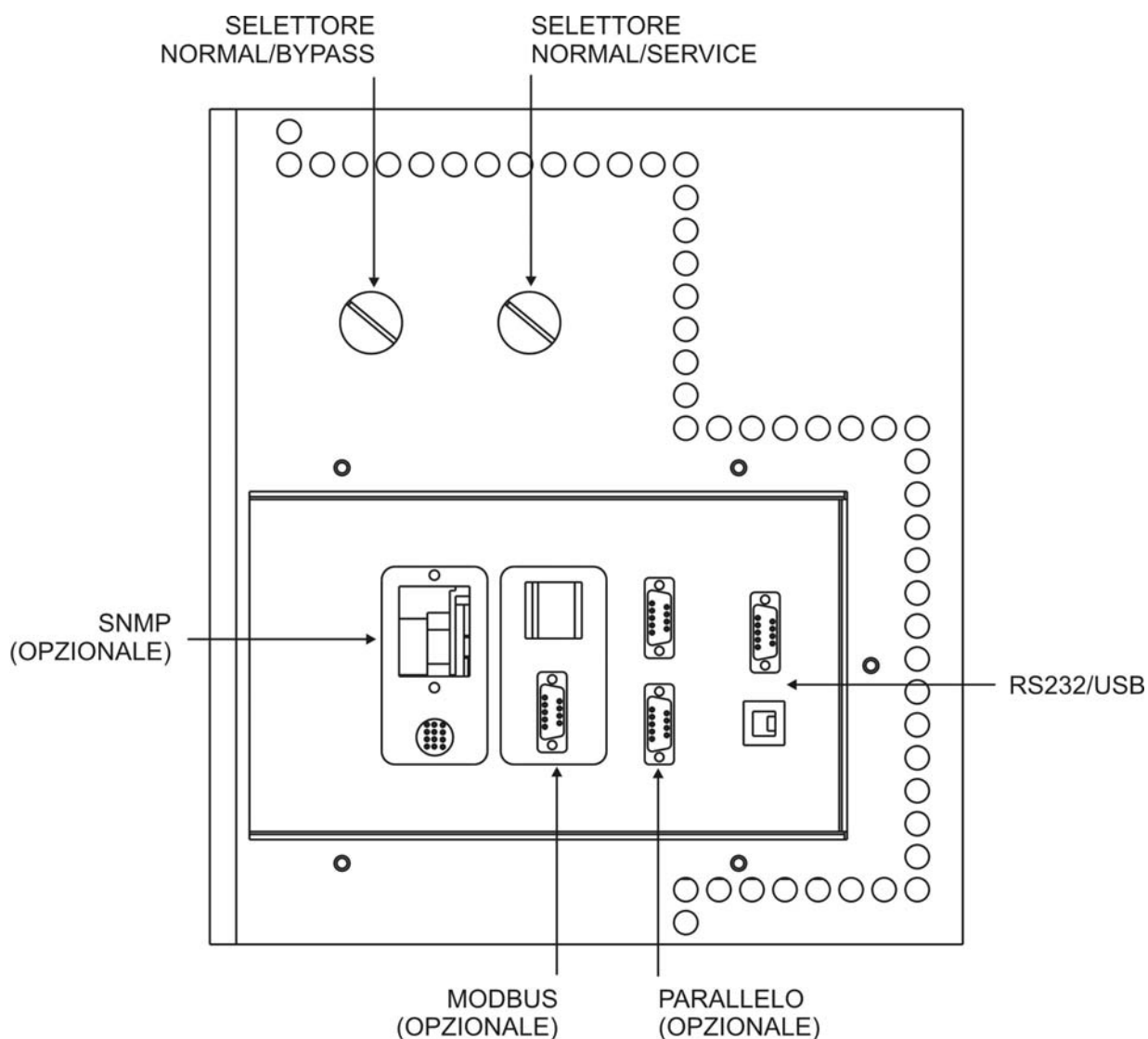
Figura 9 – Interfacce KEOR HP
