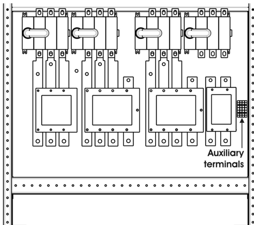
Illustration 7 – Position des bornes auxiliaires du KEOR HP
