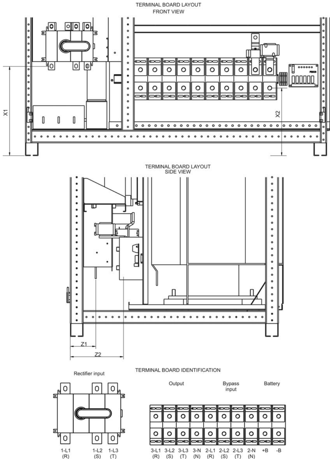
Illustration 6 – Position des bornes du KEOR HP
