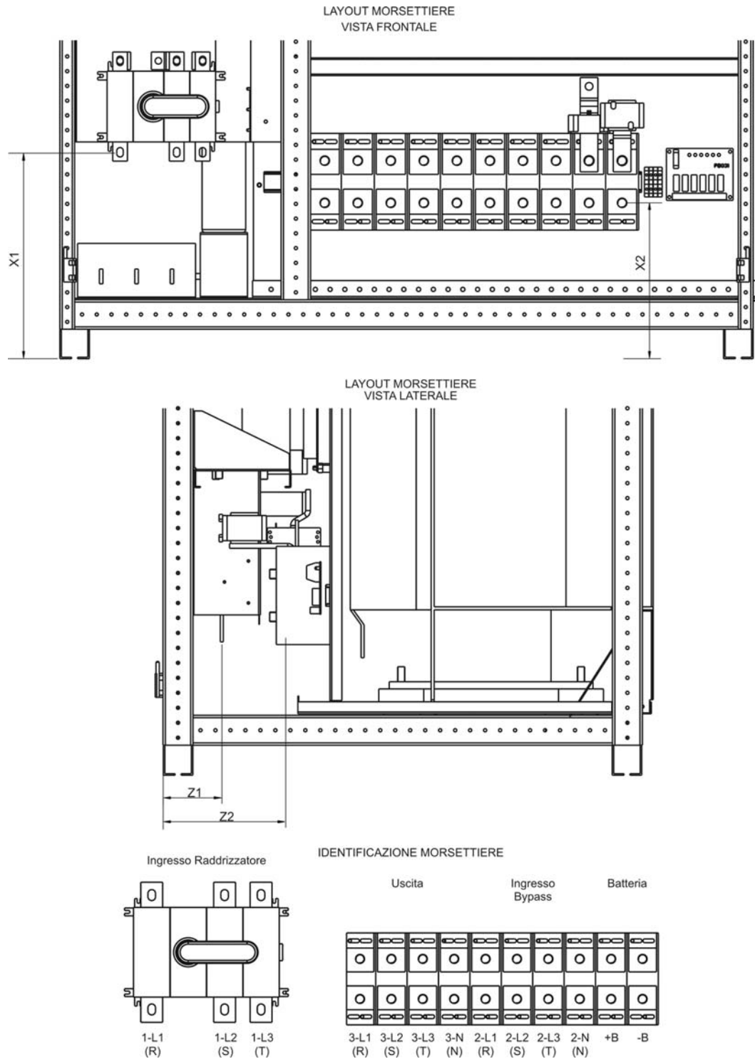
Figura 6 – Posizione morsetti potenza KEOR HP
