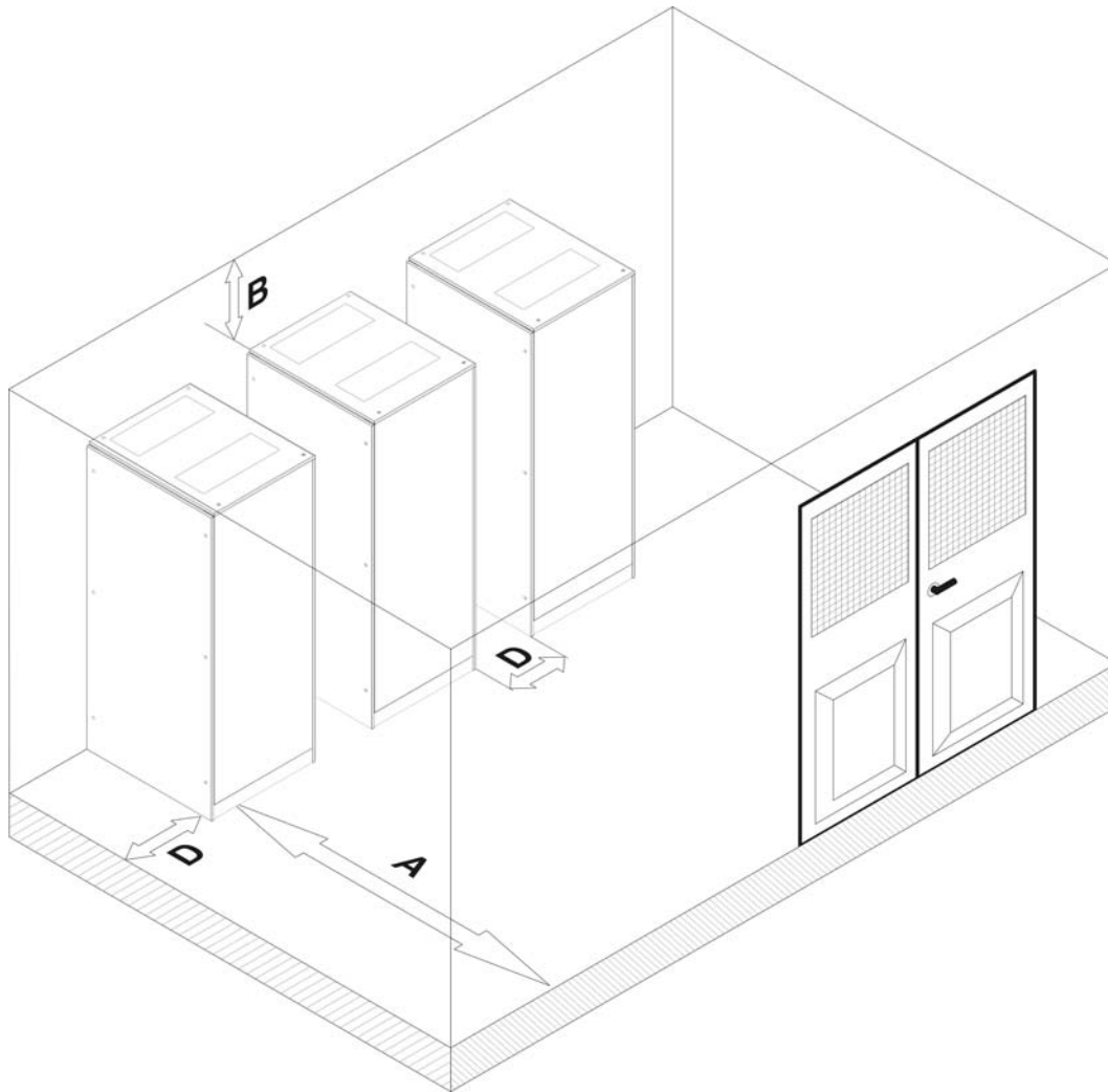
Illustration 5 – Dégagement minimum
